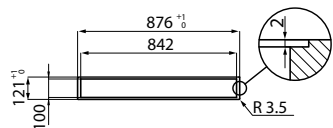
Foro per installazione filotop
