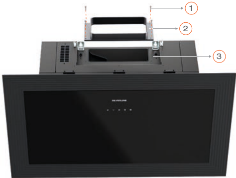
Utilizzo Alternativo in Forma Aspirante Fig 2
