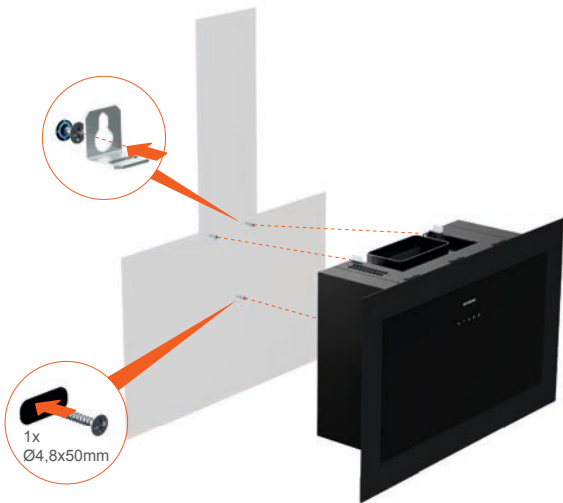
Fig 5 Schema Installazione Preparare la Cappa
