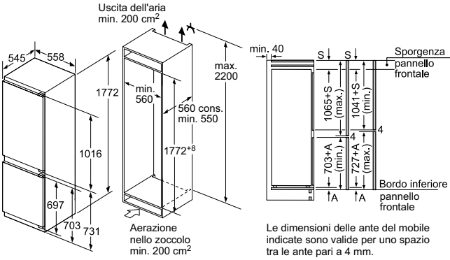
Consiglio per la distanza per cerniera piatta
