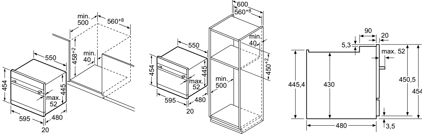
Dimensioni in mm.
