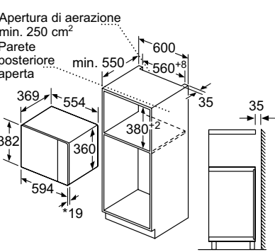
INCASSO A SEMI COLONNA
