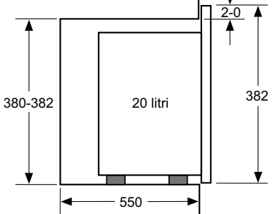
PROIEZIONE LATERALE
