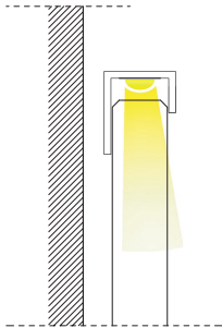
ILLUMINAZIONE LED INTEGRATA
