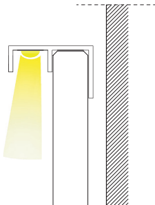
ILLUMINAZIONE LED RADENTE GRAZING LED LIGHTING
