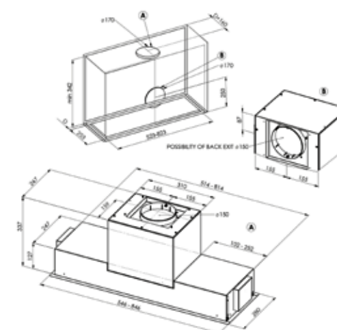
Schemi dimensionali e di installazione
