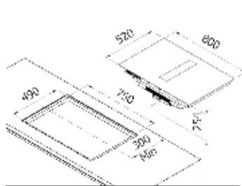
Installazione sopratop
