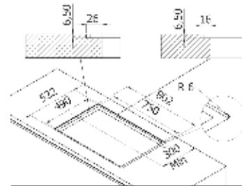
Installazione a filotop
