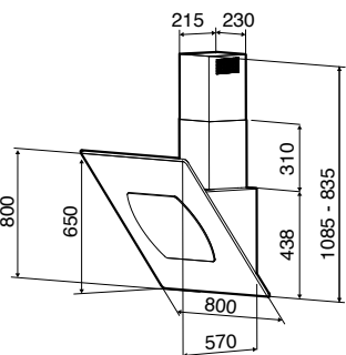
Schemi dimensionali e di installazione
