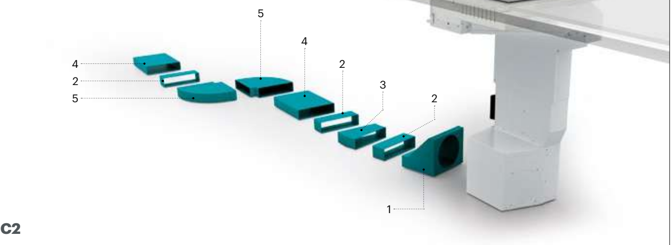
INSTALLAZIONE IN MOBILI CON ZOCCOLO H=6cm Riferimento accessori pag. 154
