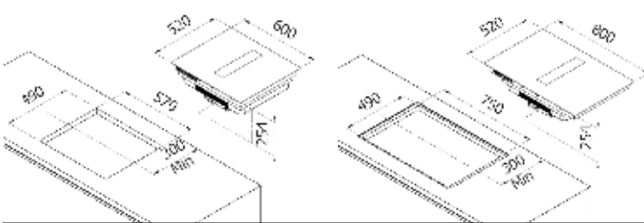
Installazione sopratop
