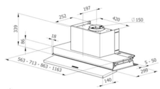
Sliver versione aspirante
