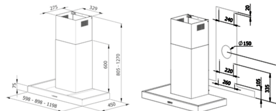
Schemi dimensionali e di installazione
