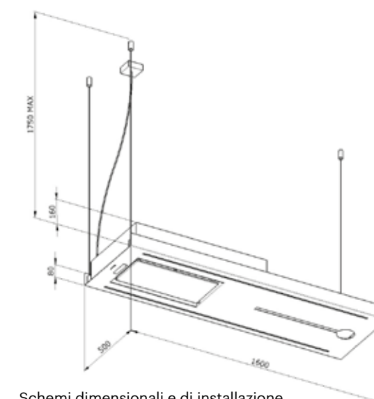
Schemi dimensionali e di installazione
