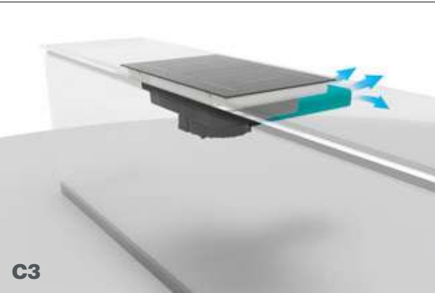
INSTALLAZIONE CON SCARICO ARIA POSTERIORE Riferimento accessori pag. 154
