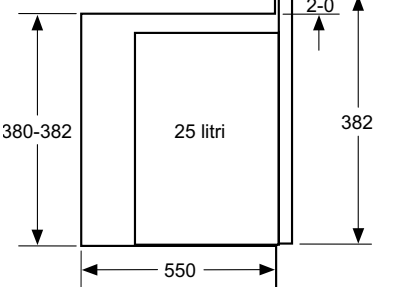
PROIEZIONE LATERALE
