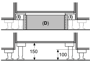
Installazione con altezza della base del mobile <150mm È necessario aumentare l'altezza dell'alloggiamento del modulo del robot a minimo 150mm.
