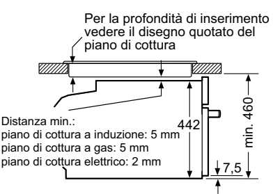
INCASSO SOTTO PIANO COTTURA
