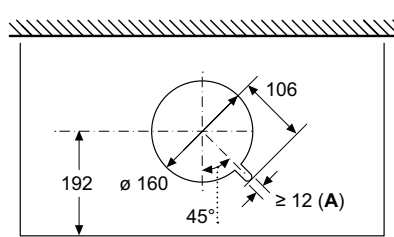
Vista dall'alto
