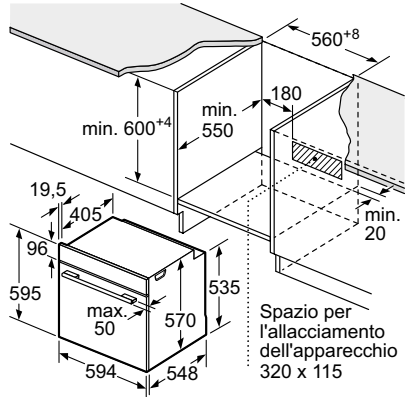
INCASSO SOTTOPIANO
