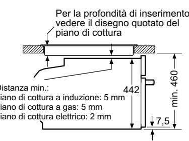
INCASSO SOTTO PIANO COTTURA
