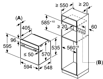
INCASSO A COLONNA
