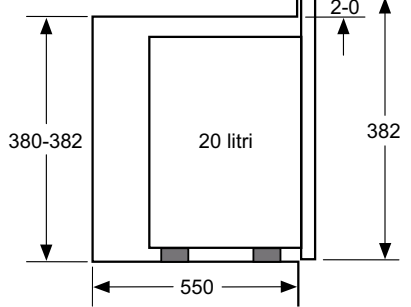
PROIEZIONE LATERALE
