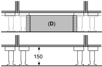
Installazione con altezza della base del mobile ≥150mm dal pavimento
