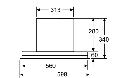
Vista frontale
