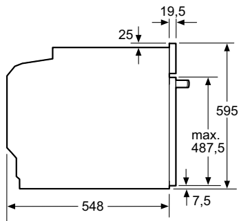
PROIEZIONE LATERALE
